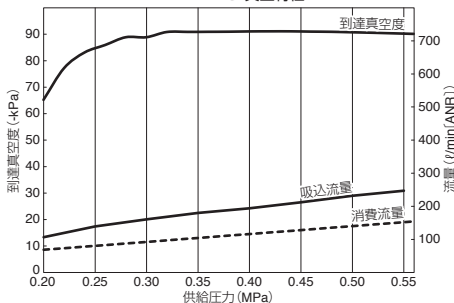
VVVE27 真空特性
