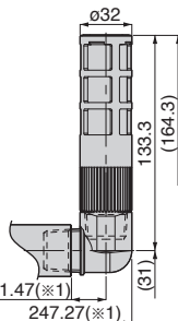
サイレンサ エルポブロック使用時
